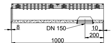
Élément avaloir
