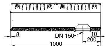
Boîte avaloir
